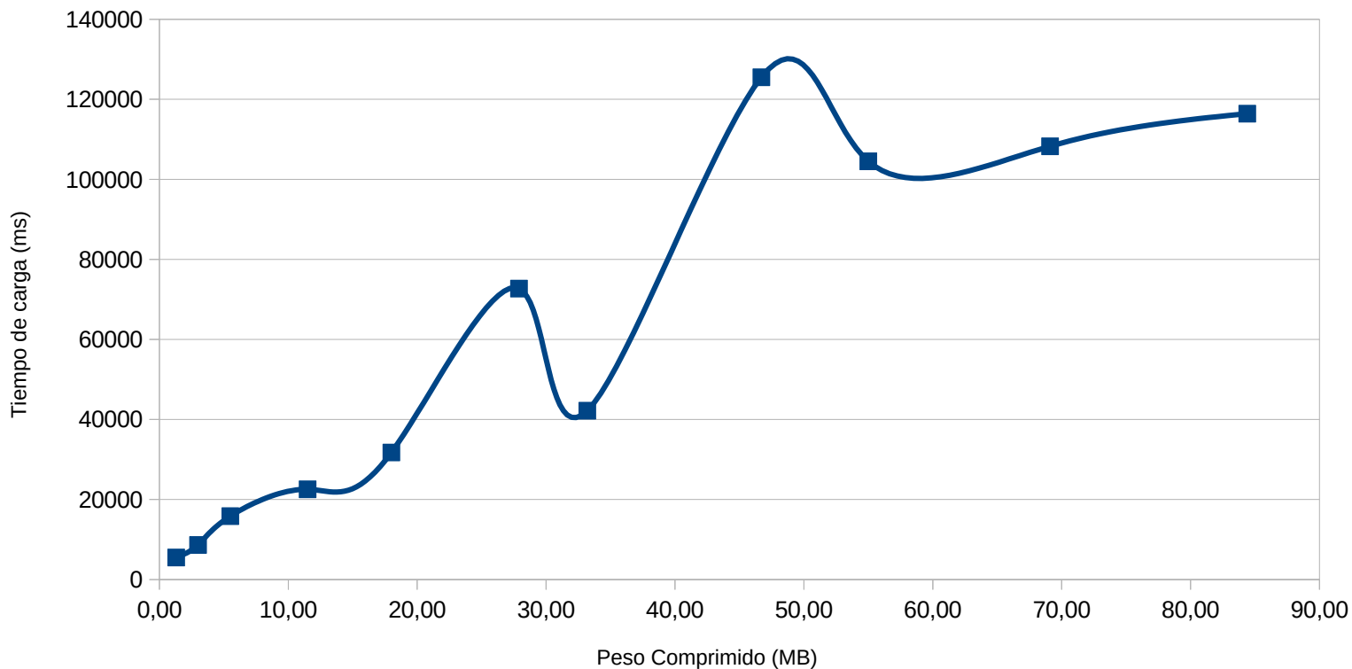
Comparativa con archivos comprimidos
