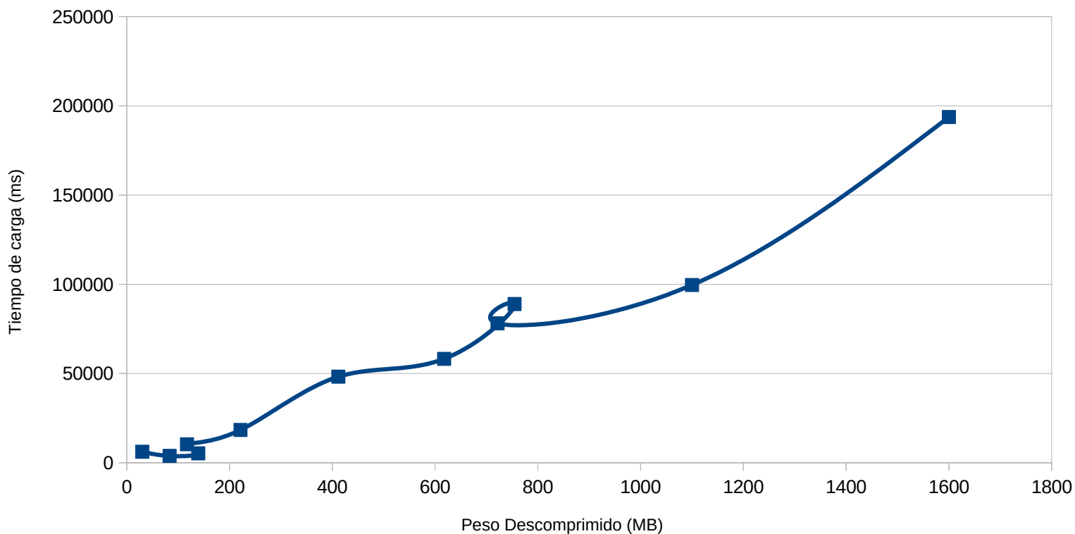
Comparativa con archivos descomprimidos
